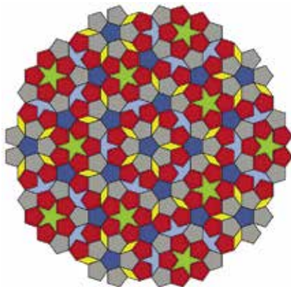
Рис. 22. Фрагмент мозаики Пенроуза
