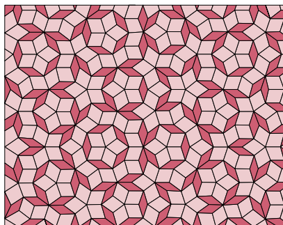
Рис. 24. Мозаика из ромбов с острыми углами 36^\circ и 72^\circ
